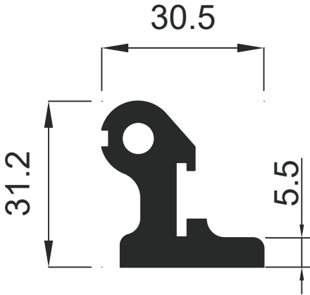
1241 1.082 Kg / m
