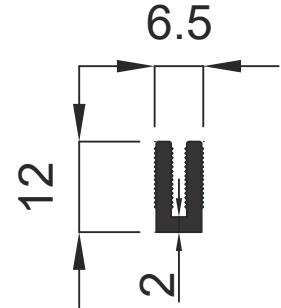
1248 0.145 Kg / m
