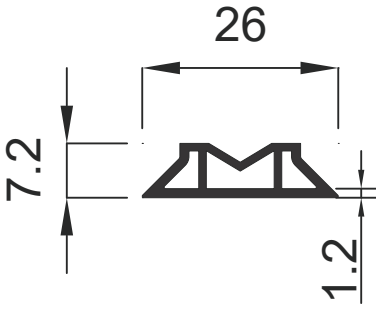
1324 0.199 Kg / m
