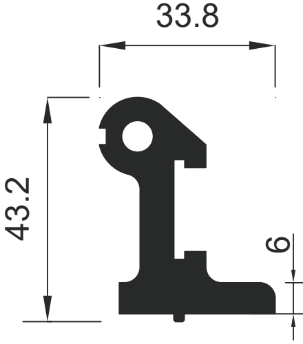
1226 1.477 Kg / m
