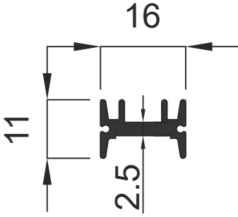
1026 0.190 Kg / m
