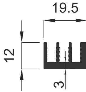
1156 0.318 Kg / m
