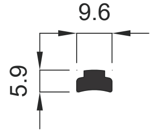
1187 0.120 Kg / m
