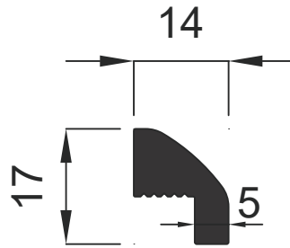
2159 0.348 Kg / m
