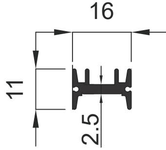
1213 0.188 Kg / m
