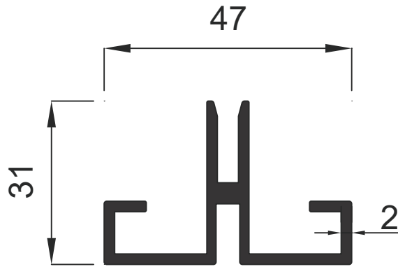
1486 0.743 Kg / m
