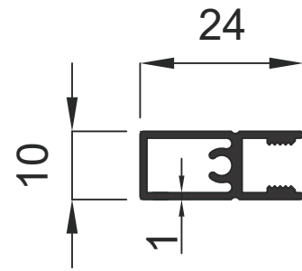
945 0.225 Kg / m
