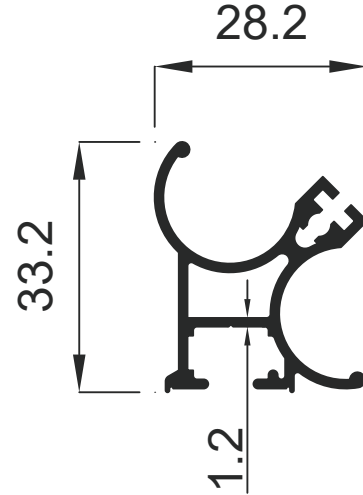
902 0.440 Kg / m
