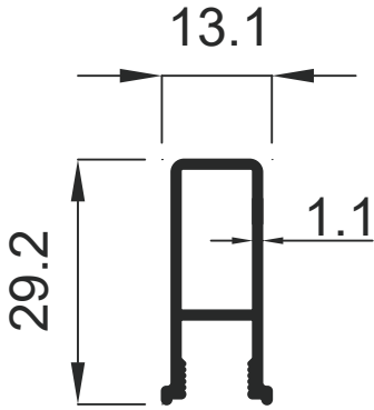
1770 0.241 Kg / m
