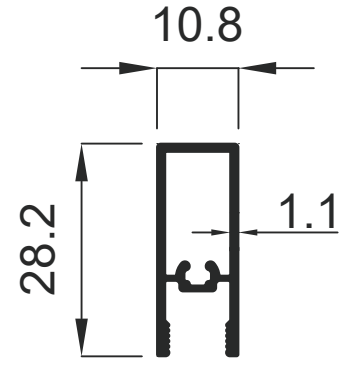
1771 0.244 Kg / m
