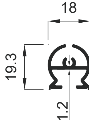
906 0.255 Kg / m
