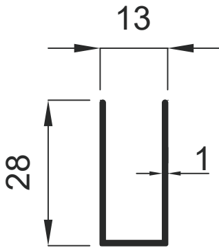
937 0.182 Kg / m
