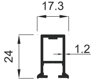
1764 0.287 Kg / m
