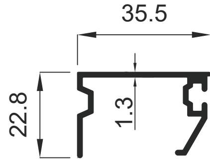
1782 0.347 Kg / m
