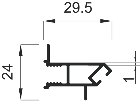
939 0.275 Kg / m
