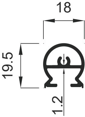
904 0.263 Kg / m
