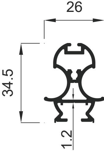
903 0.494 Kg / m
