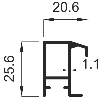
1769 0.290 Kg / m
