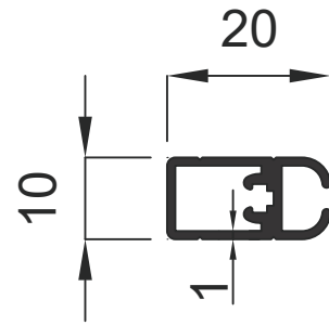
930 0.196 Kg / m
