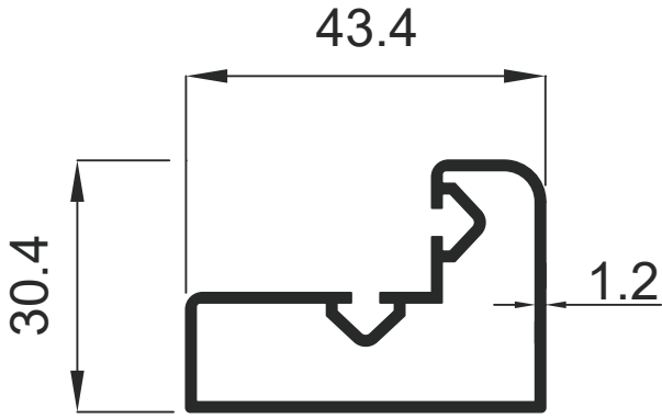
1932 0.518 Kg / m
