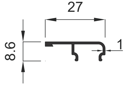
1037 0.128 Kg / m
